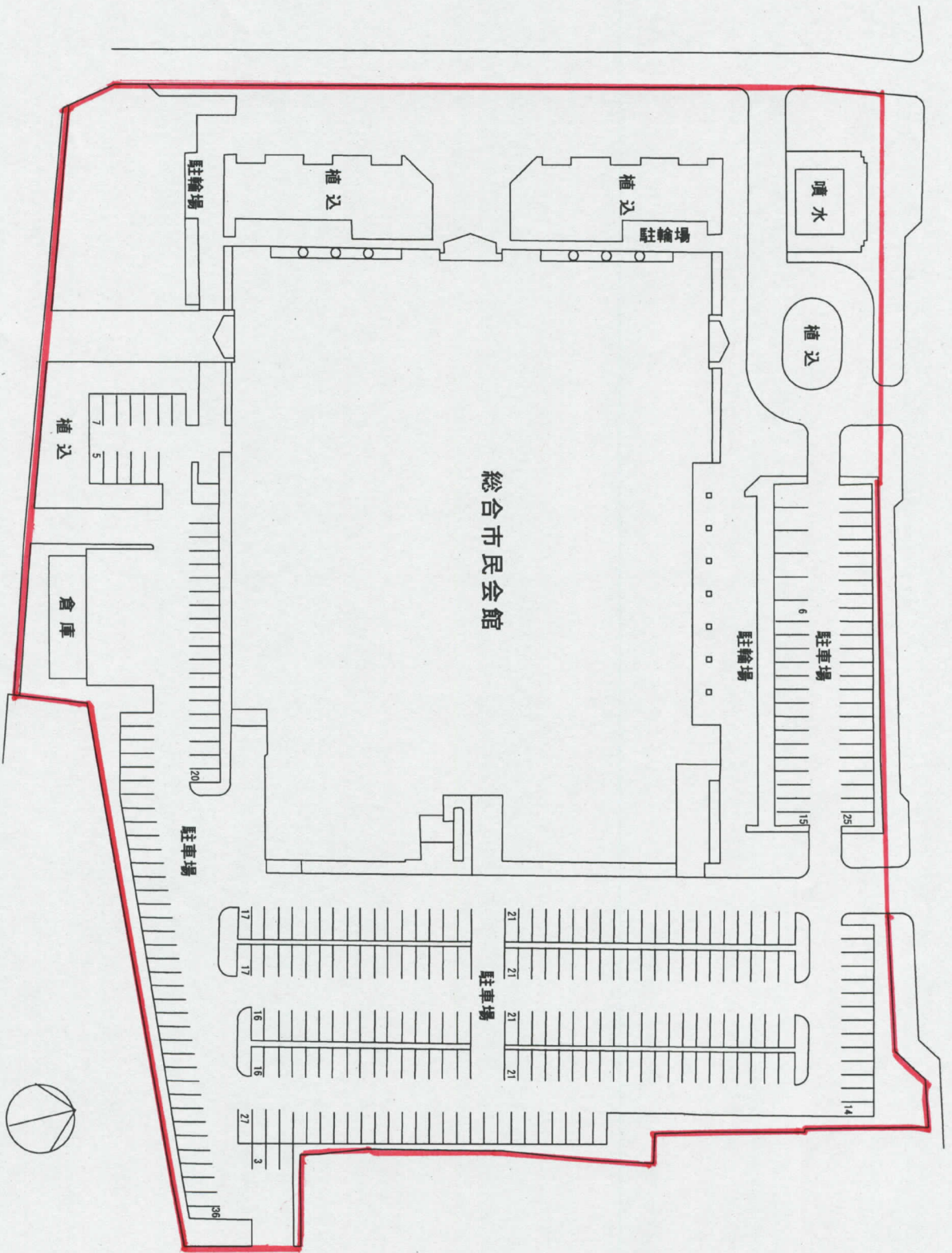
総合市民会館 配置図
