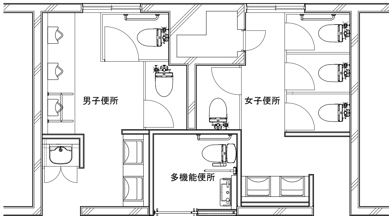
改修後 1 階平面図
