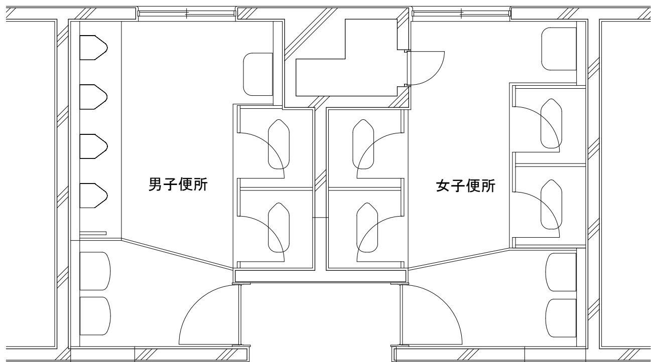
既存 1 階平面図
