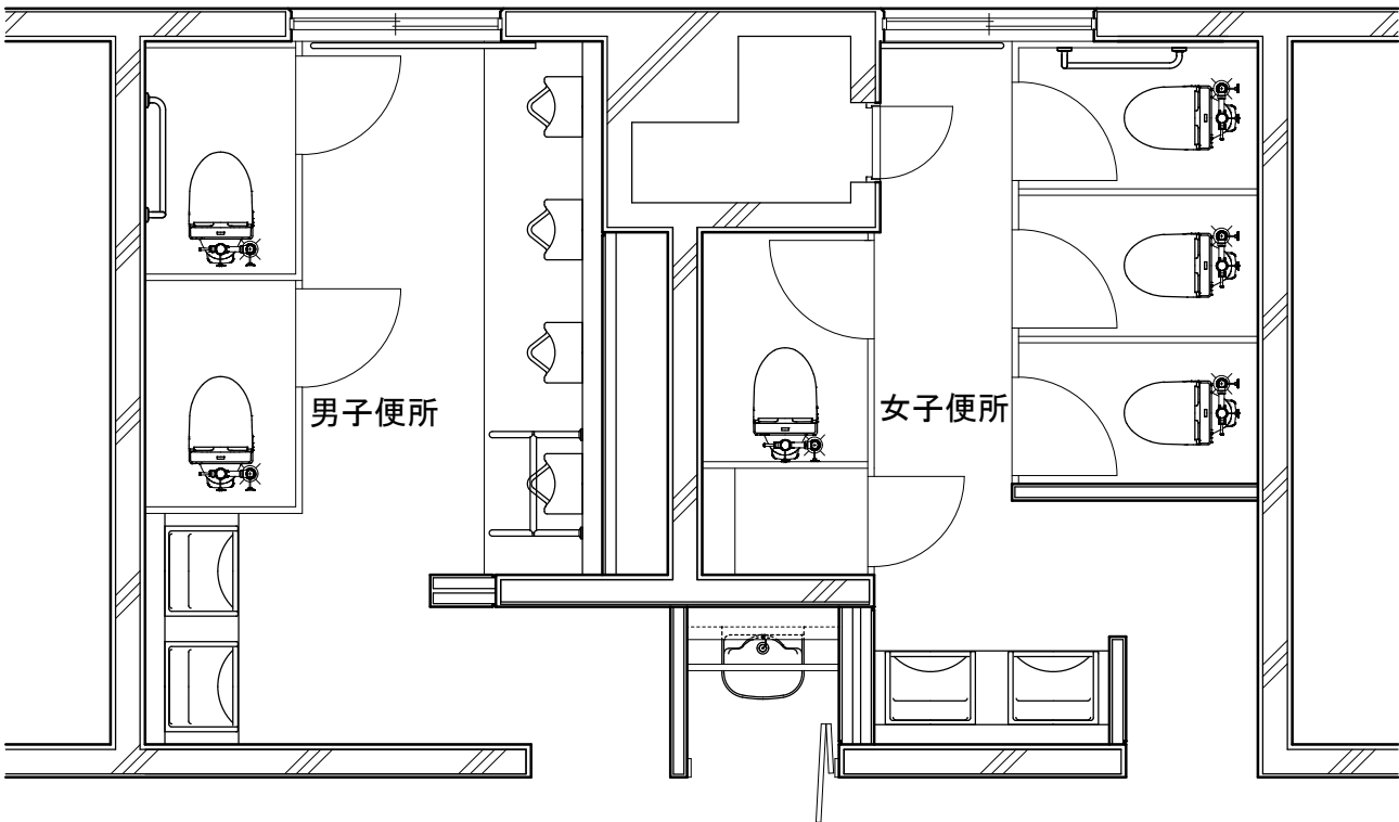
改修後 2、3階平面図
