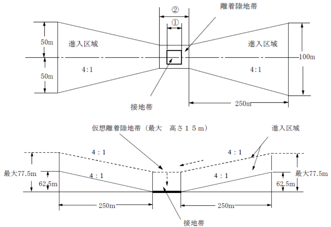
平面図
