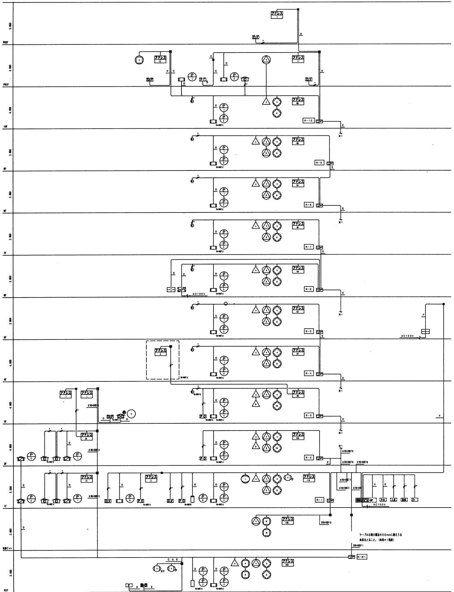
設備系統図
