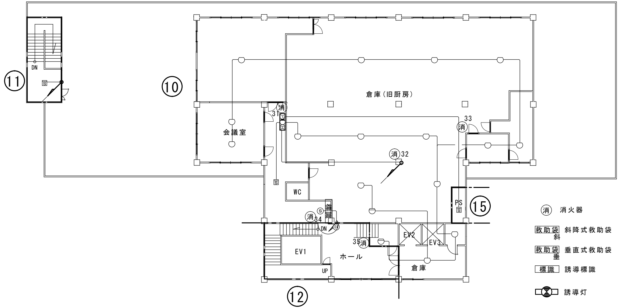
5 階平面図
