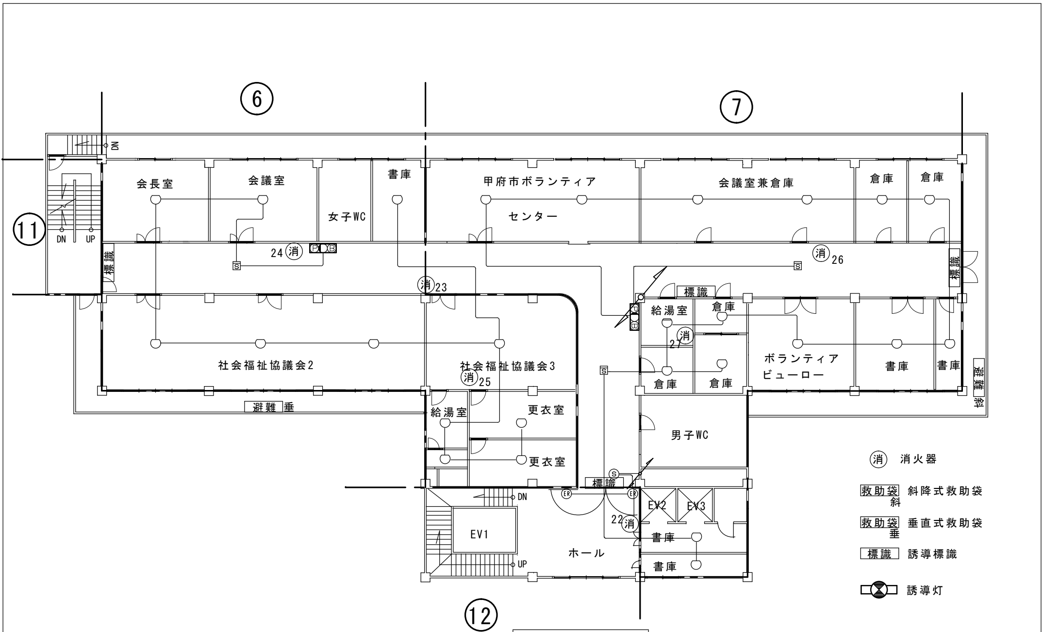
3階平面図
