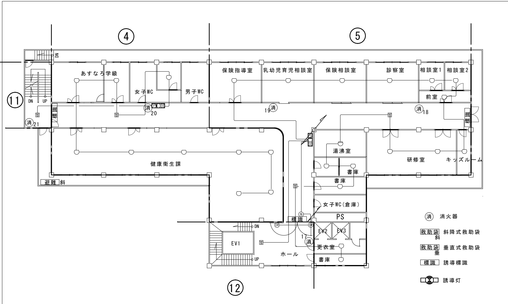
2階平面図
