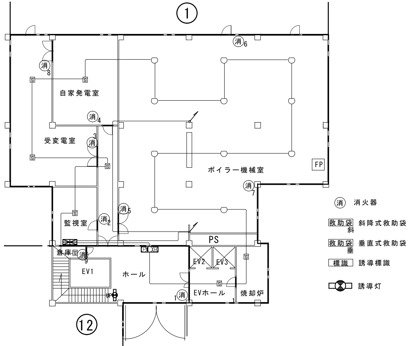
BF1平面図
