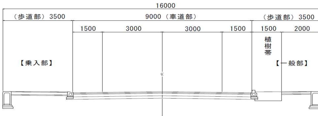
標準断面図
